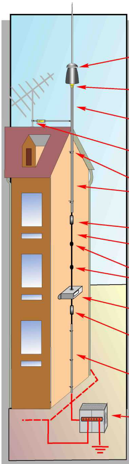
Obr. 10 Instalace jímacího systému nimbus
